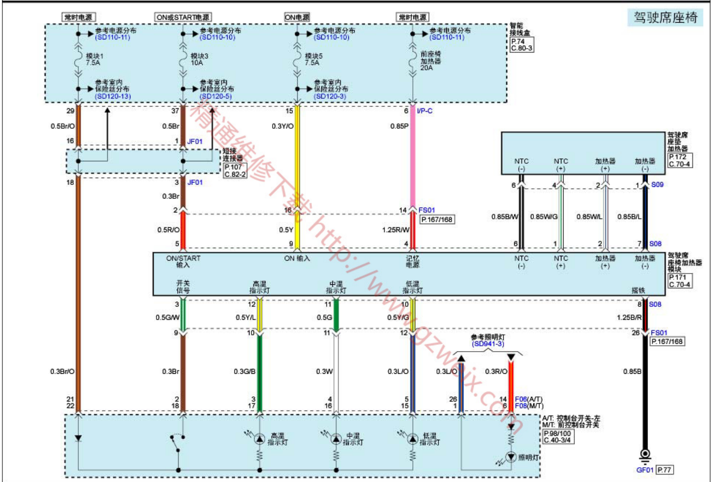
座椅加热器(1)
